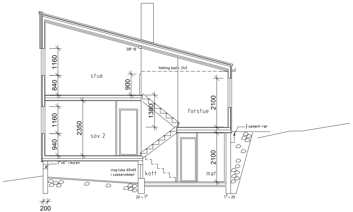
snitt B-B
